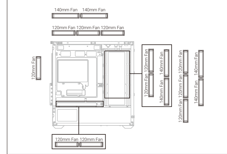
Fan Support
