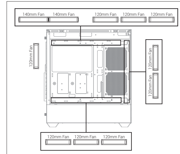
(6a) Install Top Fan
