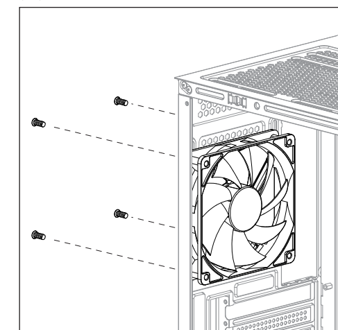
(6d) Install Rear Fan
