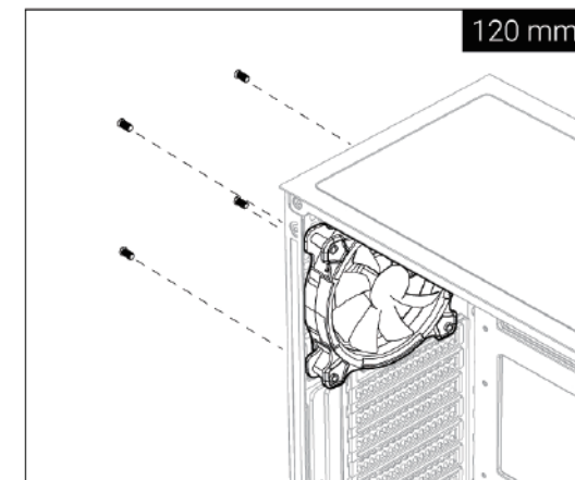
(6c) Install Rear Fan
