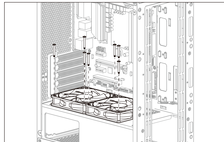
(7) Install PSU Fan
